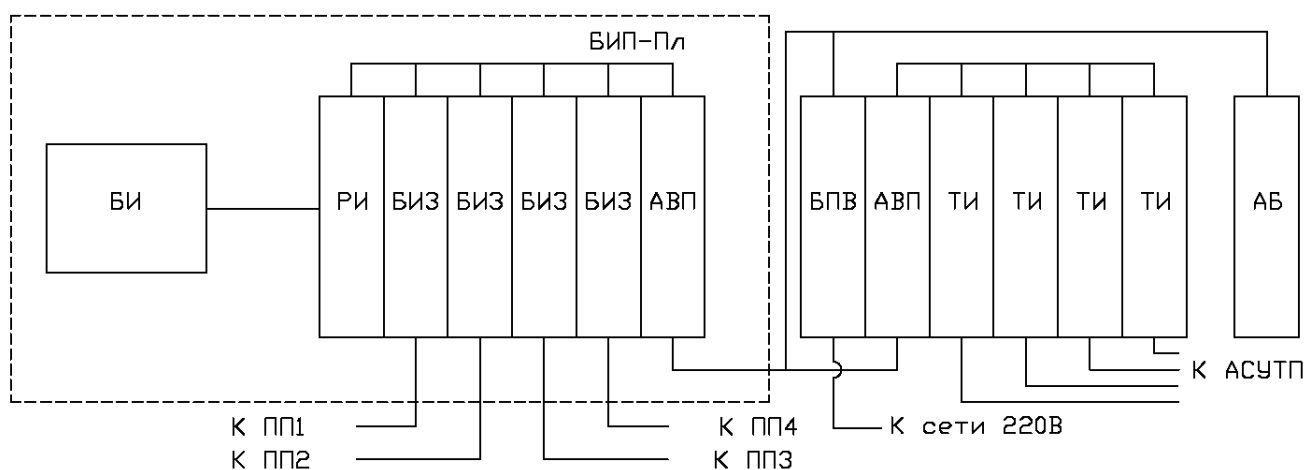
д). Трех- четырехканальный ВИП ИРВИС-РС4М с ТИ по каждому каналу
